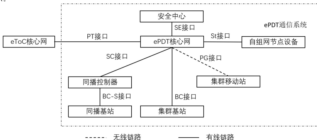
图 1 应急专用数字集群 (ePDT) 通信系统网络架构图
