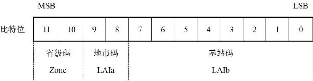
图 2 无线位置识别号 LAI 结构图
