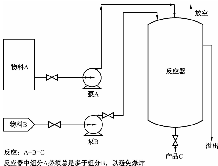
图 B.1 简化流程
