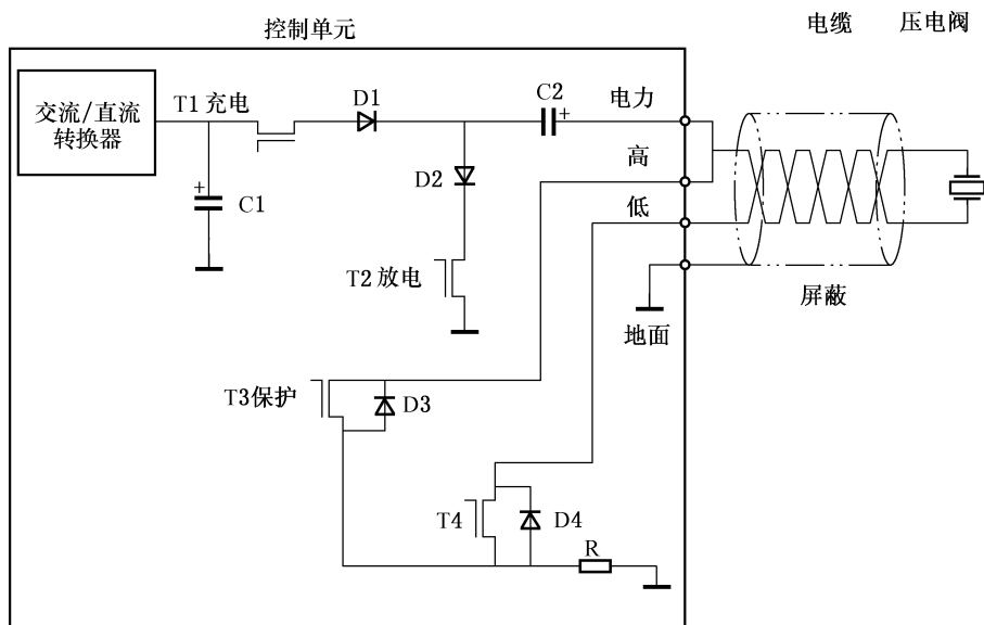
图 B.3 压电阀控制系统
