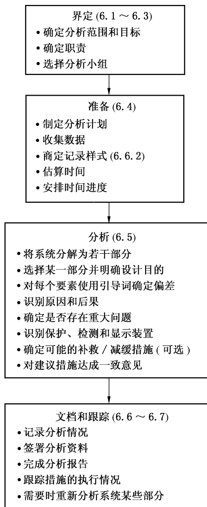
图 1 HAZOP 分析程序
