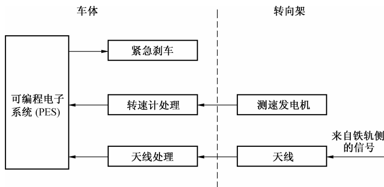
图 B.2 车载 ATP 设备
