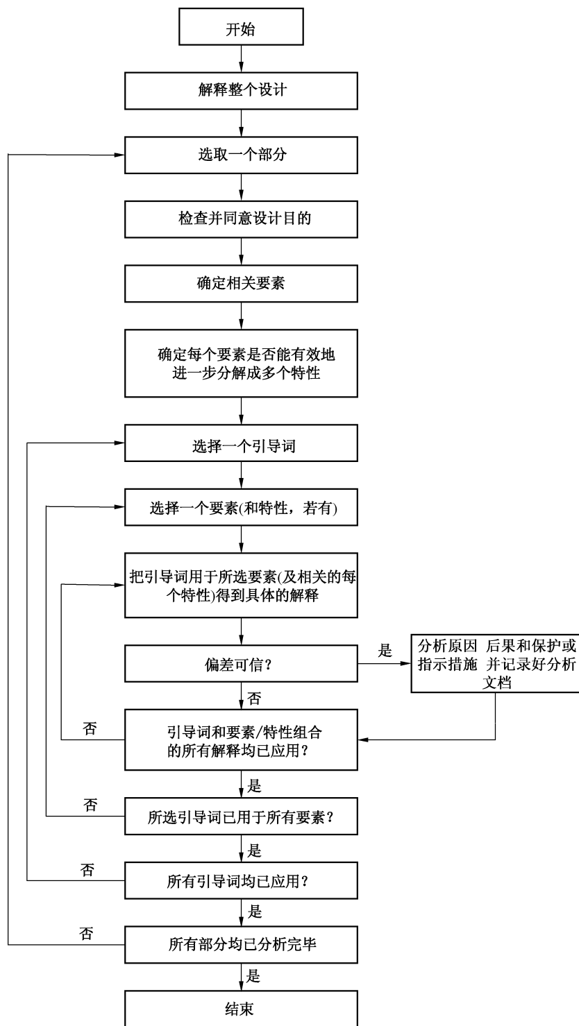
图 3 HAZOP 分析程序流程——引导词优先顺序
