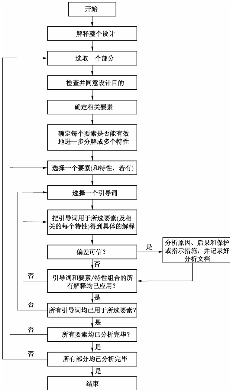
图 2 HAZOP 分析程序流程——要素优先顺序
