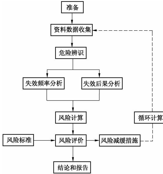
图 A.1 定量风险评价基本程序
