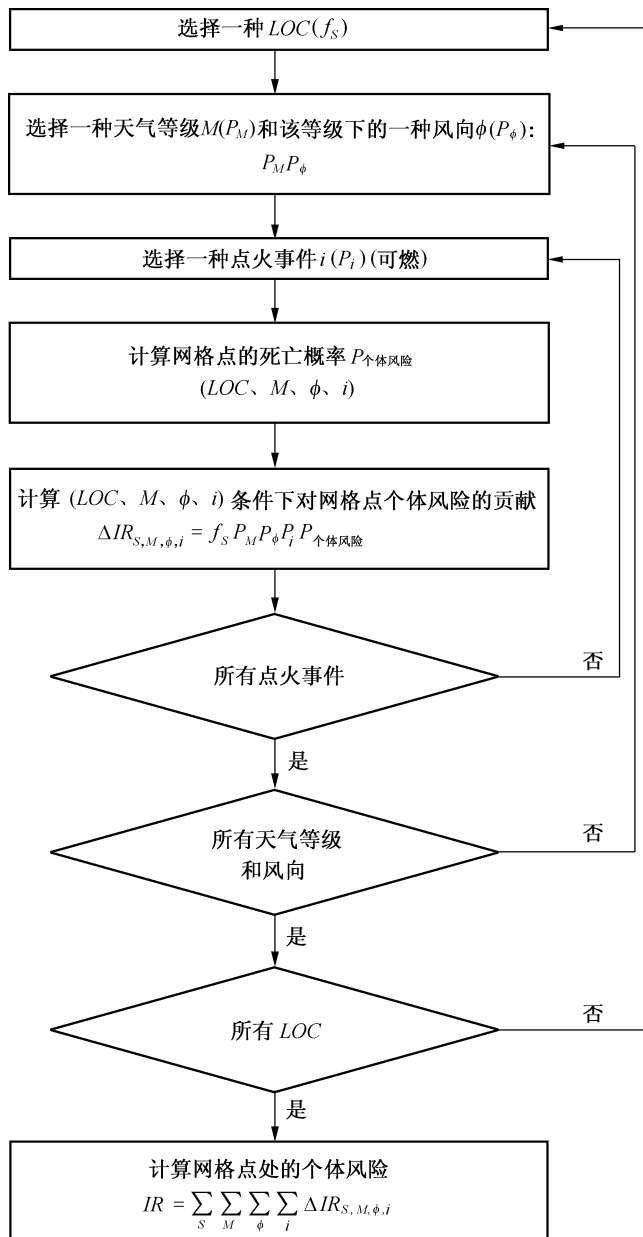
图 1 网格点处的个体风险计算程序
